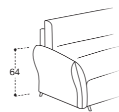
BRACCIOLO 1 L. 16 CM H. 64 CM
