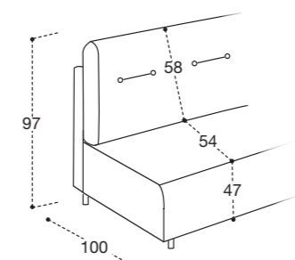
SCocca 2,5 POSTI 142 Materasso-Mattress-Matelas 120 x 193 x 18
